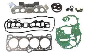
واشر کامل موتور Gasket Kit , Engine Overhaul P.N: 0701011009
